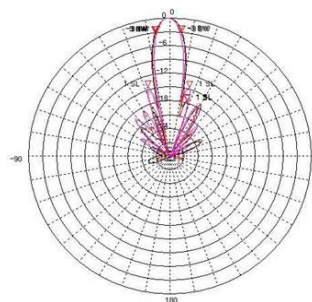
0°Tilt
