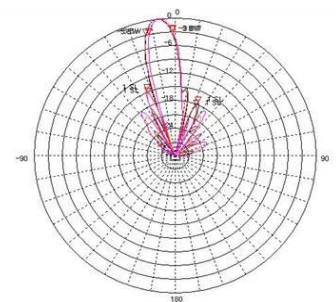
6°Tilt
