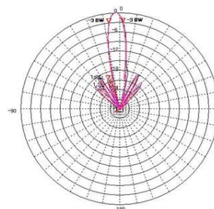
2°Tilt
