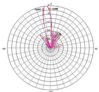
6°Tilt
